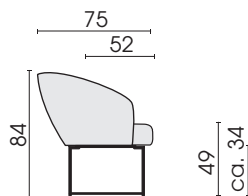
Seitenansicht Typ 146
